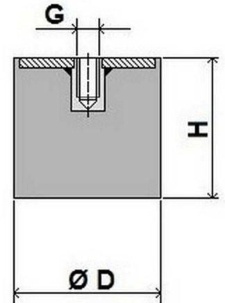
PIEDINO-FEMMINA
