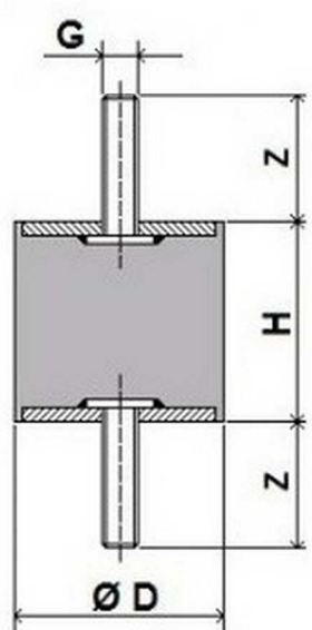
MASCHIO-MASCHIO
