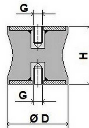
SGOLATO F-F
