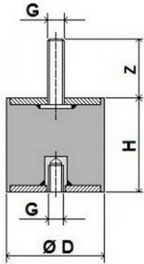
MASCHIO-FEMMINA
