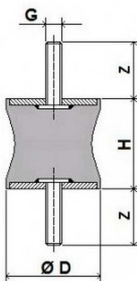
SGOLATO M-M
