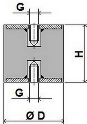
FEMMINA-FEMMINA
