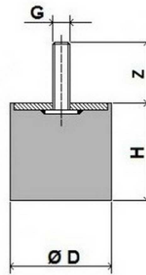
PIEDINO-MASCHIO
